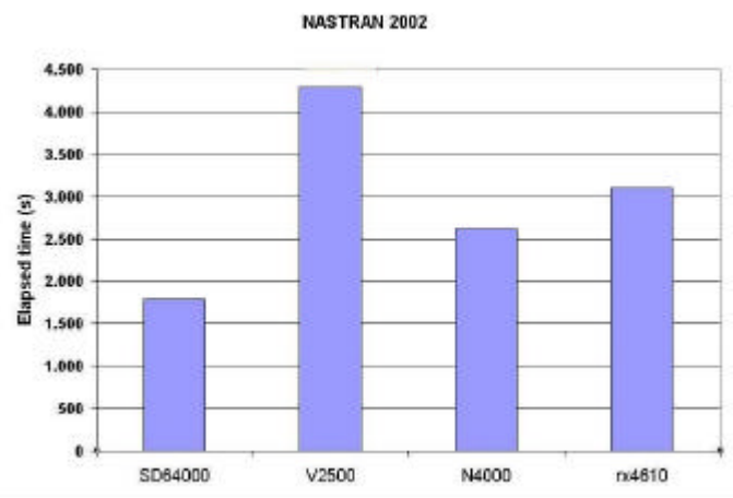
Fig. 2 - Tempi di esecuzione per caso benchmark monoprocesso di NASTRAN 2002
