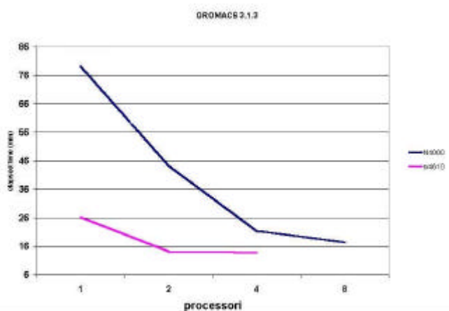
Fig.4 - Confronto tra N4000 e rx4610 al variare del numero di CPU per un test GROMACS.
